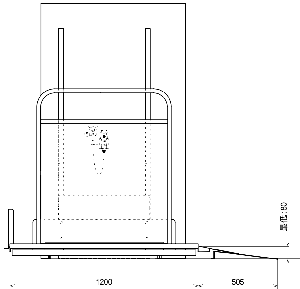
全体構造据付図 (DA-100)
